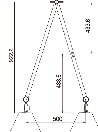
使用寸法図（500mm に開いている時）
