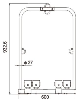
外寸法図（閉じている時）
