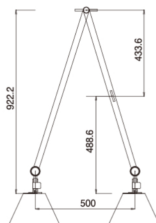
使用寸法図（500mm に開いている時）
