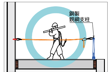
(C) クランプ⇄鋼製親綱支柱
