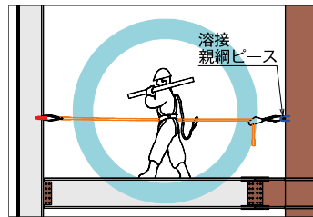
(B) クランプ⇄溶接親綱ピース
