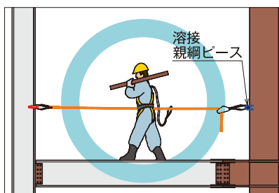
(B) クランプ⇄溶接親綱ピース
